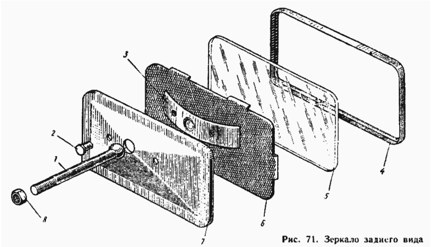
Рис. 71. Зеркало заднего вида.
